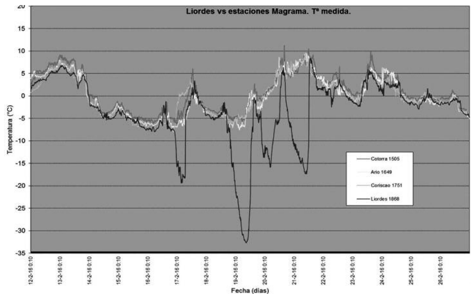
Gráfica comparativa del descenso de temperatura. Agrupación Jous Picos de E.
